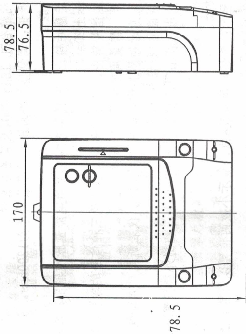
仪表外形图
