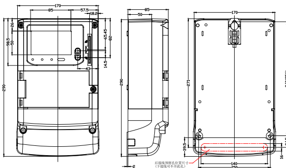
图 1: 安装尺寸图
