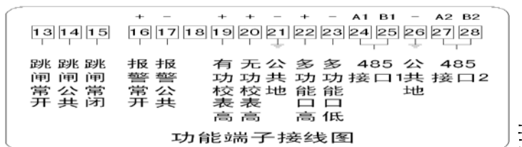
图 3：辅助端子排列图
