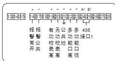
内置 RS485 表功能端子
