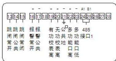
外置 RS485 表功能端子
