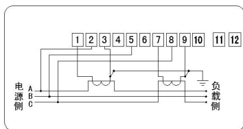
三相三线经电流互感器接入式接线图
