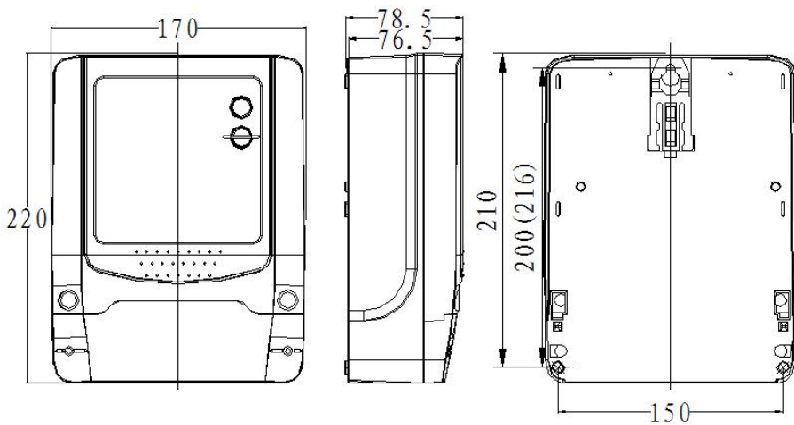
外形与安装图
