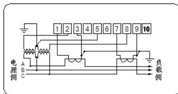
三相三线经电压、电流互感器接入式接线图
