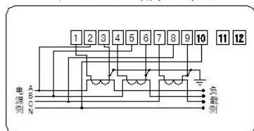
三相四线经电流互感器接入式接线图
