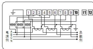
三相四线经电压、电流互感器接入式接线图
