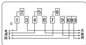
三相四线直接接入式接线图
